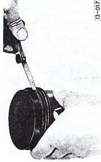
Fig. 9 Segments de piston : vérification du jeu en hauteur
