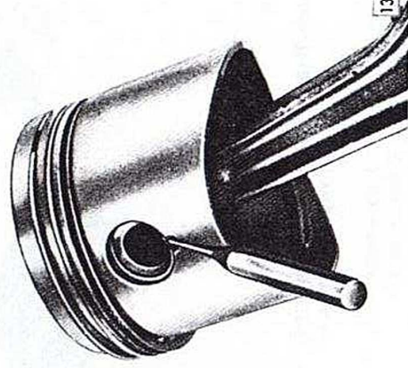
Fig. 4 Segment d'arrêt : extraction en faisant lever
