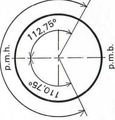
ÉPURE DE DISTRIBUTION pour une levée des soupapes de 1,5 mm
