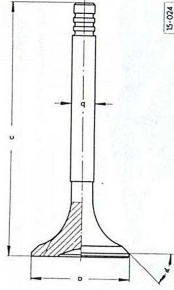
Fig. 6 Cote des soupapes
