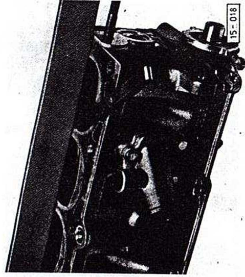
Fig. 1 Culasse : vérification du gauchissement
