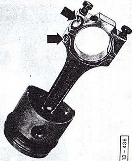
Fig. 3 Bielle : position de montage
