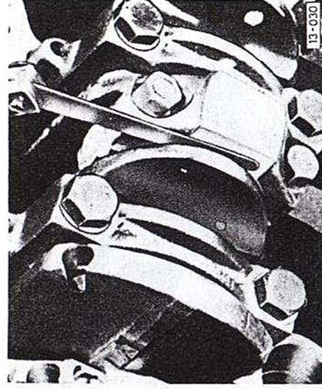
Fig. 13 Bielle : vérification du jeu axial
