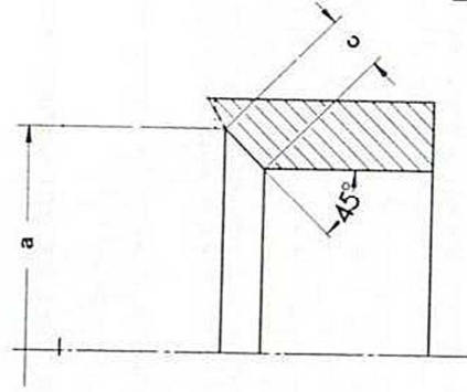
Fig. 9 Siège de soupape d'échappement : rectification
