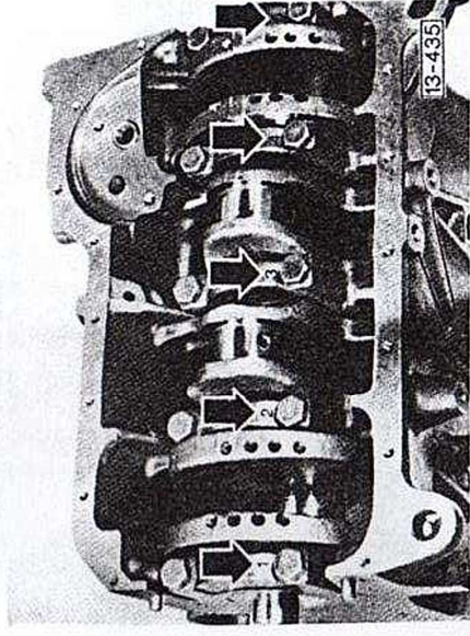
Fig. 6 Vilebrequin - chapeaux de paliers : position de montage
