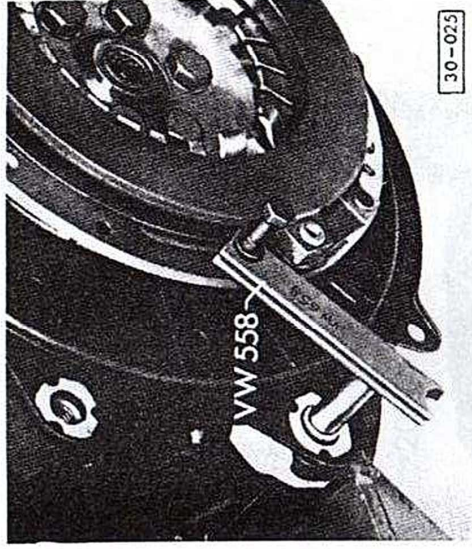
Fig. 4 Plateau de pression : dépose et repose
