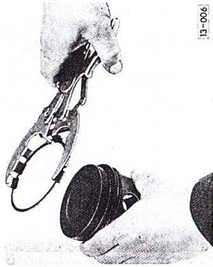
Fig. 7 Segments de piston : dépose et repose
