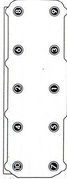
Fig. 2 Culasse : dépôt et repose
