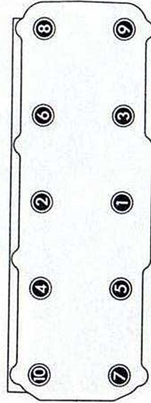
Fig. 1 Flaque d'étanchéité AV avec protection de la courroie crantée : dépose et repose
