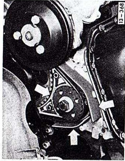
Fig. 1 Flaque d'étanchéité AV avec protection de la courroie crantée : dépose et repose
