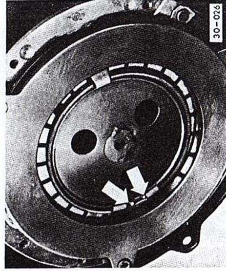
Fig. 3 Bague d'arrêt : repose Tenir compte de la position des extrémités
