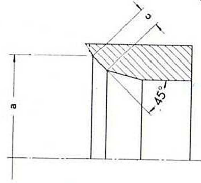
Fig. 8 Siège de soupape d'admission : rectification
